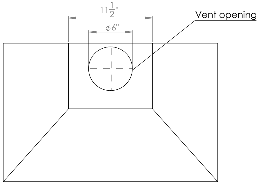
TOP
